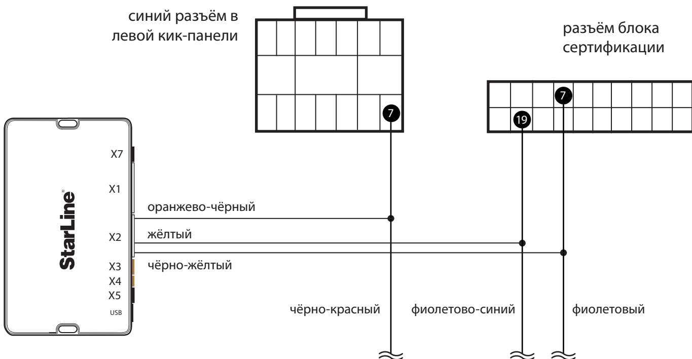
Схема 1. Подключение цепей автозапуска двигателя
