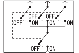
REAR DOOR SWITCH (LH) (E-14)
