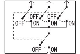
REAR DOOR SWITCH (RH) (E-07)
