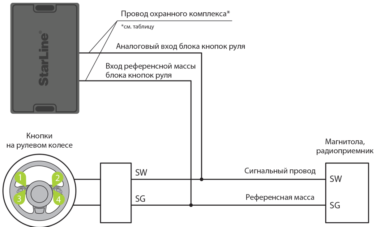
Схема подключения аналоговых кнопок
