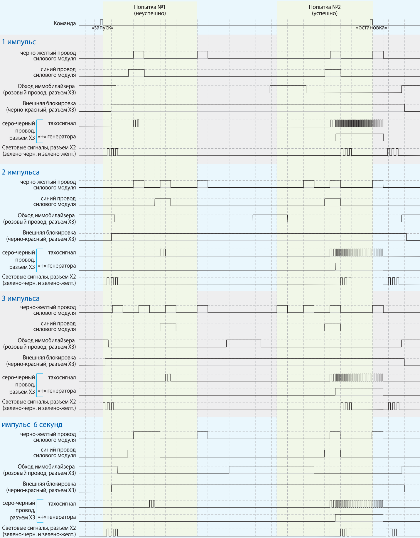
Временные диаграммы работы комплекса при дистанционном запуске двигателя в автомобилях с кнопкой «Старт/Стоп»
