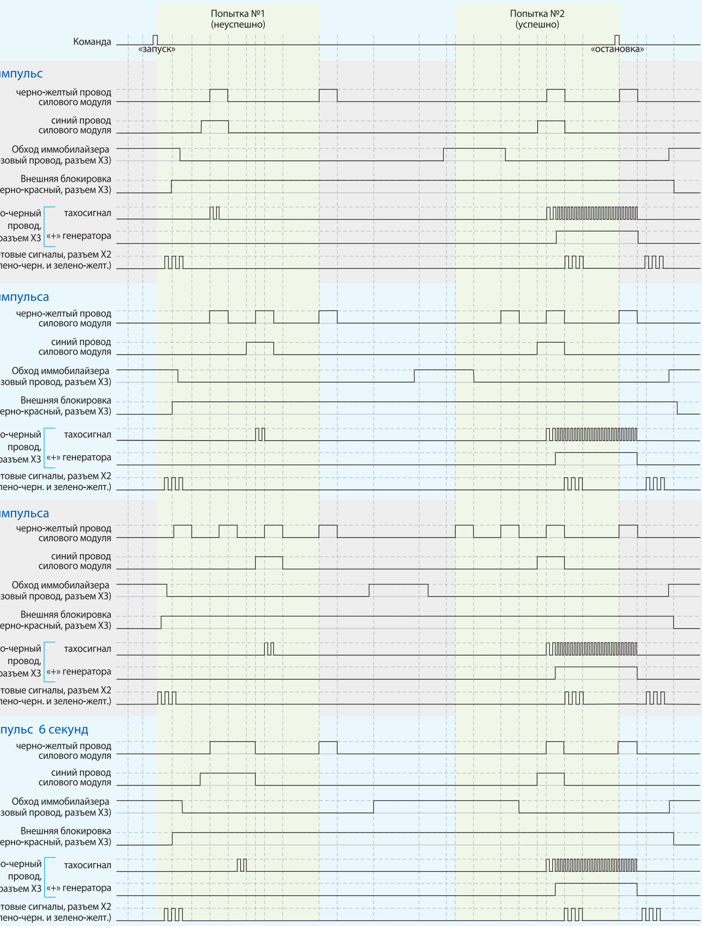
Временные диаграммы работы комплекса при дистанционном запуске двигателя в автомобилях с кнопкой «Старт/Стоп»
