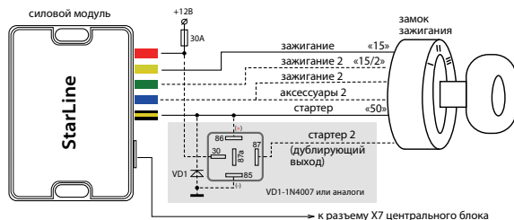
разъем X7 (слаботочные выходы)
