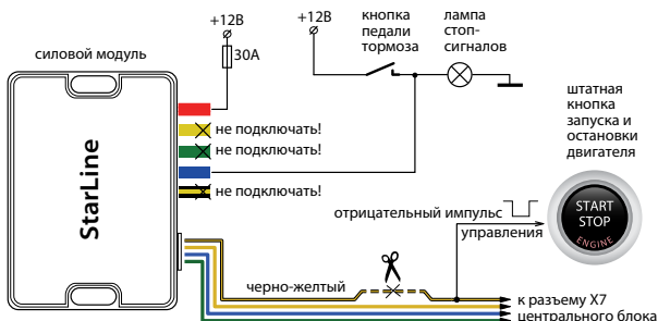
Схема 2: слаботочное управление кнопкой «старт-стоп»
