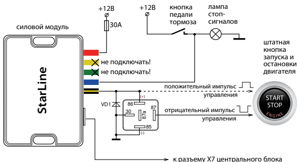
Схема 2: слаботочное управление кнопкой «старт-стоп»
