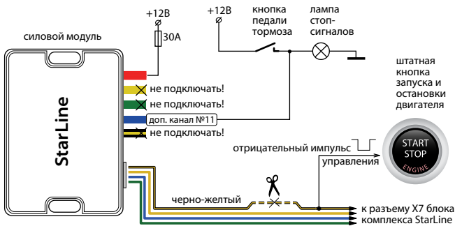
Схема 2: слаботочное управление кнопкой «старт-стоп»
