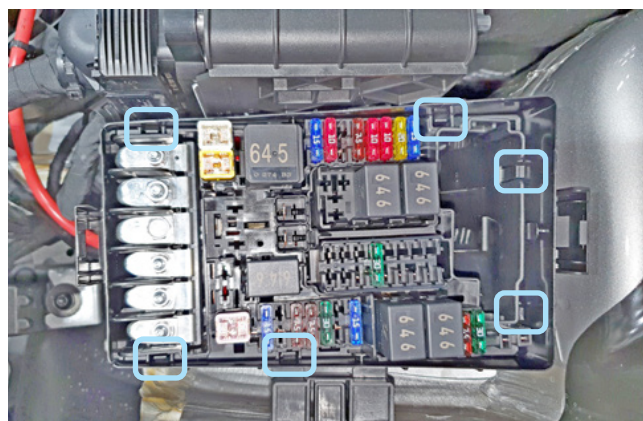
Фото 3.14. Защёлки крепления монтажного блока предохранителей
