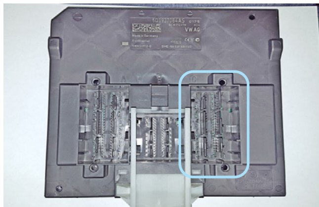
Фото 3.2. Местоположение разъёма C на блоке BCM
