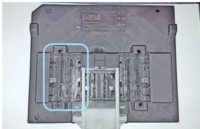
Фото 3.4. Местоположение разъёма A на блоке BCM
