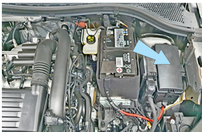
Фото 3.13. Местоположение монтажного блока предохранителей под капотом
