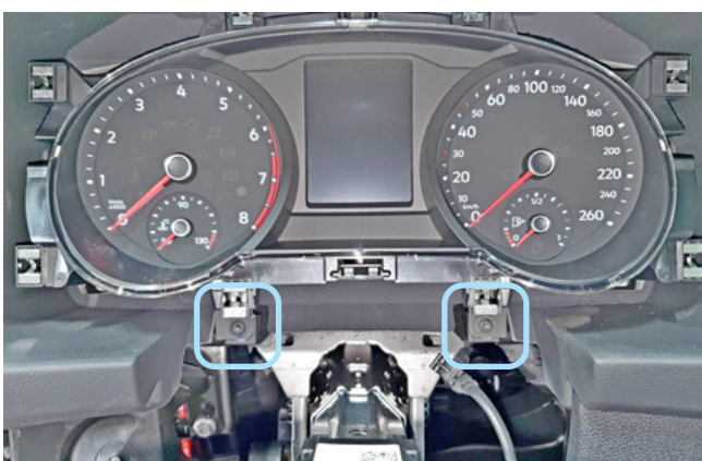
Фото 1.17. Накладка снята. Саморезы крепления панели приборов
