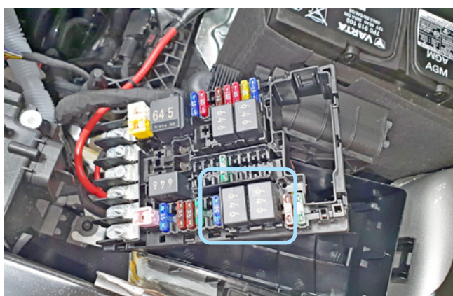
Фото 3.15. Местоположение реле управления стартером
