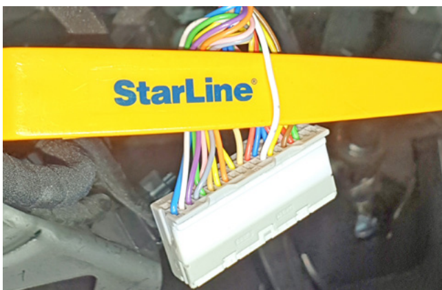
Фото 3.9. Зажигание 2 (белый)
