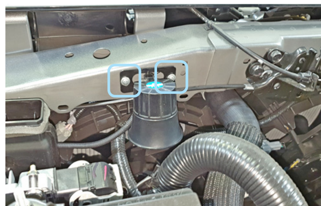
Фото 2.5. Крепление сирены
