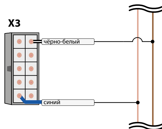
Фото 3.13. Схема подключения ЦЗ
