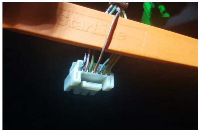
Фото 3.3. Шина CAN-A (розовый)
