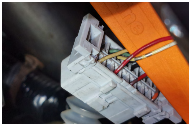
Фото 3.5. Шина CAN-B (белый и красный)
