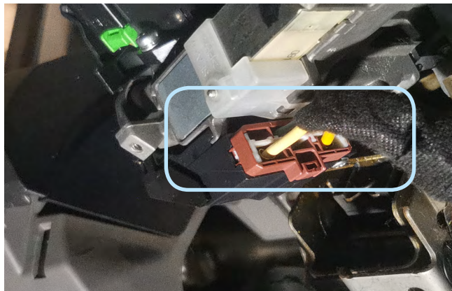
Фото 3.18. Местоположение разъёма
