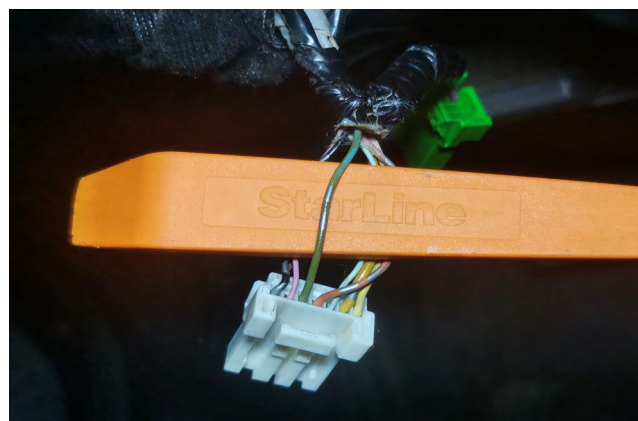
Фото 3.17. Шина данных штатного иммобилайзера (зелёный)
