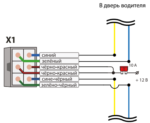
Фото 3.9. Схема подключения ЦЗ
