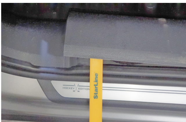
Фото 1.15. Частично снять пластиковую накладку порога двери водителя
