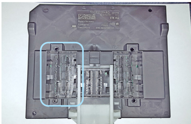
Фото 3.11. Местоположение разъёма А на блоке BCM
