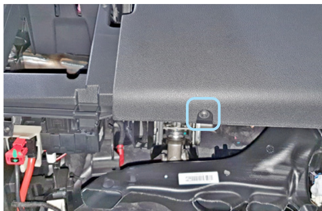
Фото 1.9. Саморез крепления в нижней части накладки
