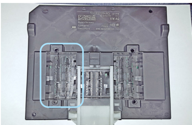
Фото 3.3. Местоположение разъёма А на блоке BCM
