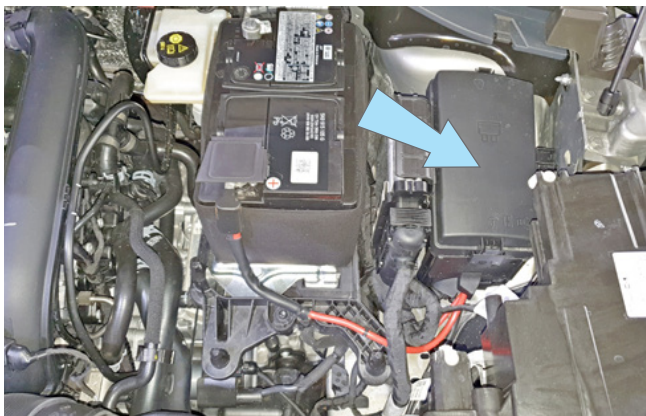
Фото 3.16. Местоположение монтажного блока предохранителей под капотом
