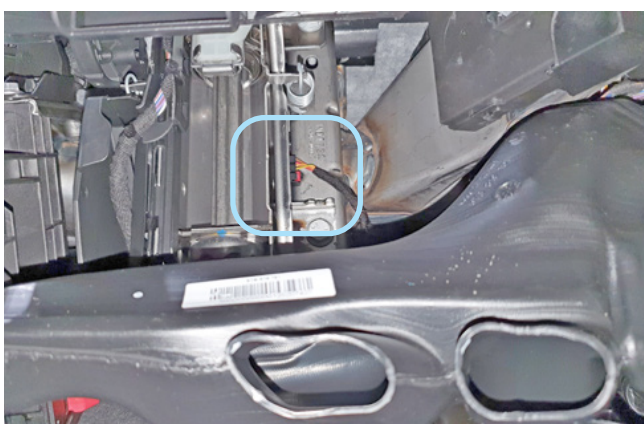
Фото 3.9. Местоположение разъёма
