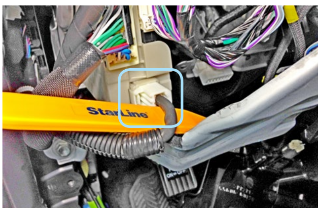
Фото 3.7. Питание +12В (чёрный)
