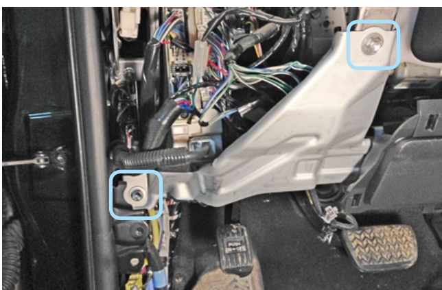
Фото 1.15. Болты крепления подушки безопасности слева
