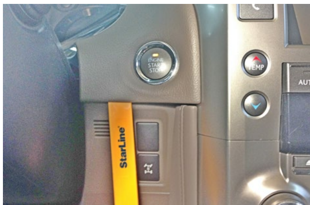
Фото 1.18. Снять накладку с кнопкой Старт-Стоп
