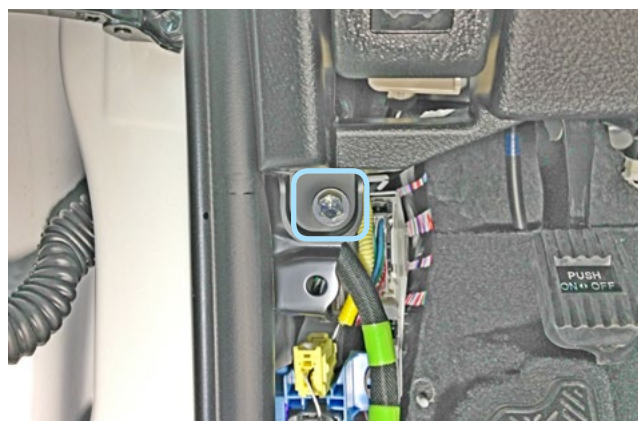
Фото 1.10. Болт крепления накладки под рулевой колонкой слева
