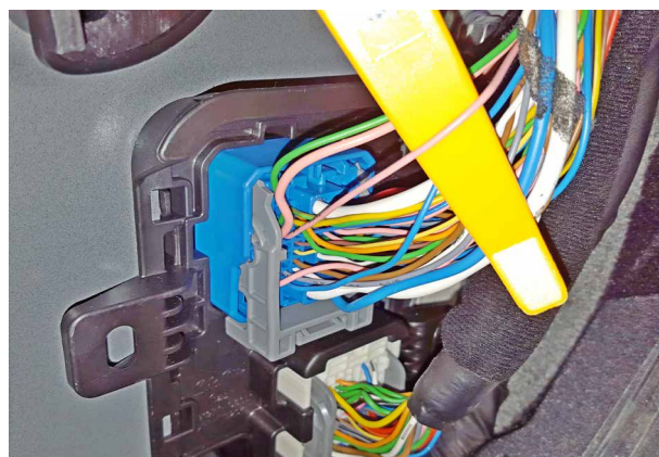
Фото 10.2. Шина данных штатного иммобилайзера (розовый)
