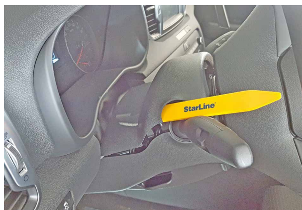
Фото 2.2. Снять верхнюю часть кожуха рулевого вала
