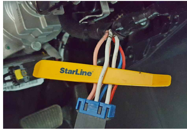
Фото 11.6. Питание +12В (белый)
