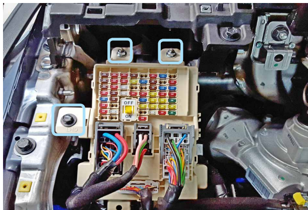
Фото 3.3. Крепление монтажного блока предохранителей
