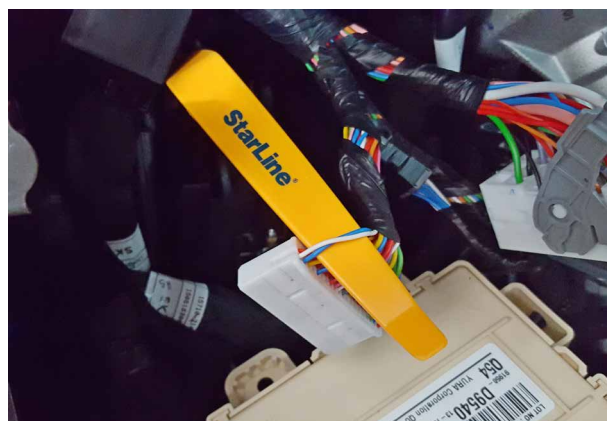
Фото 8.2. CAN-шина (синий и белый)
