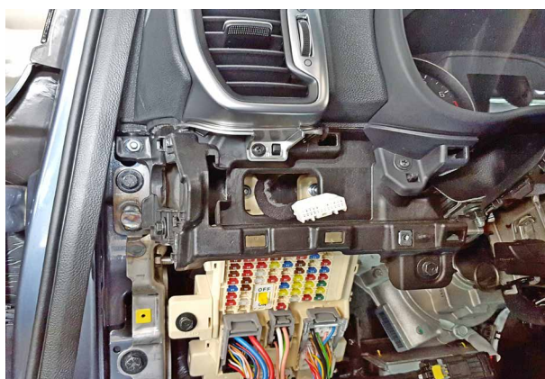
Фото 3.2. Блок кнопок снят
