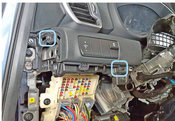
Фото 3.1. Саморезы крепления блока кнопок
