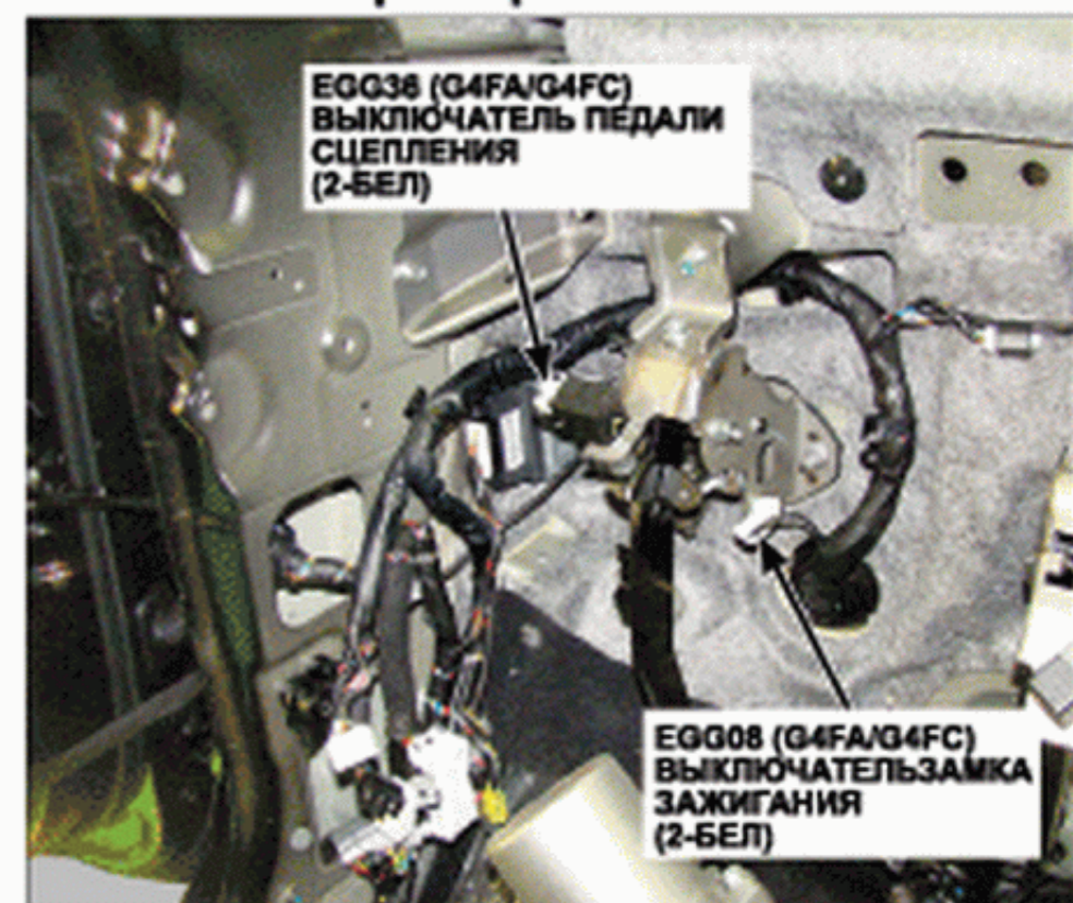
48. Задняя левая часть панели приборов
