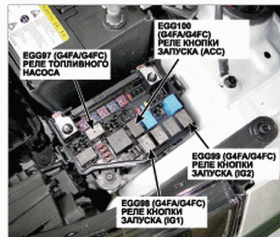
12. Левая сторона моторного отсека
