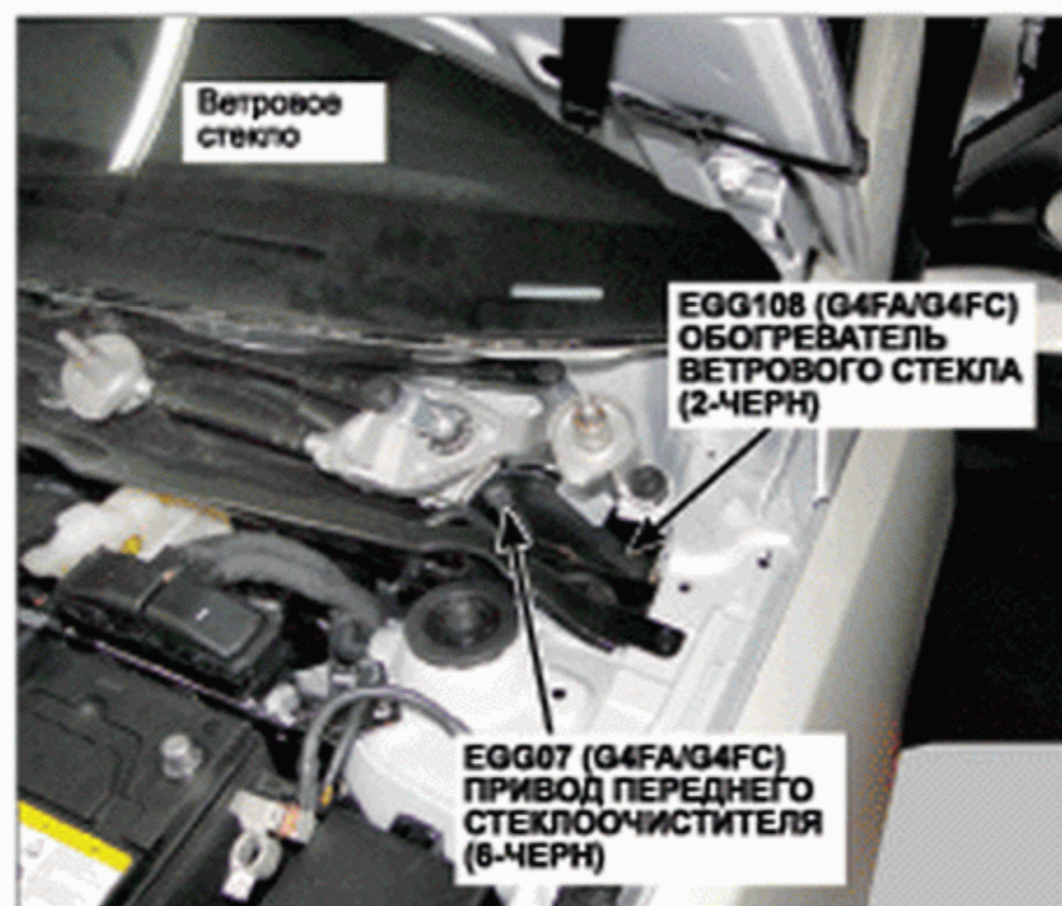
14. Левая сторона верхней панели капота
