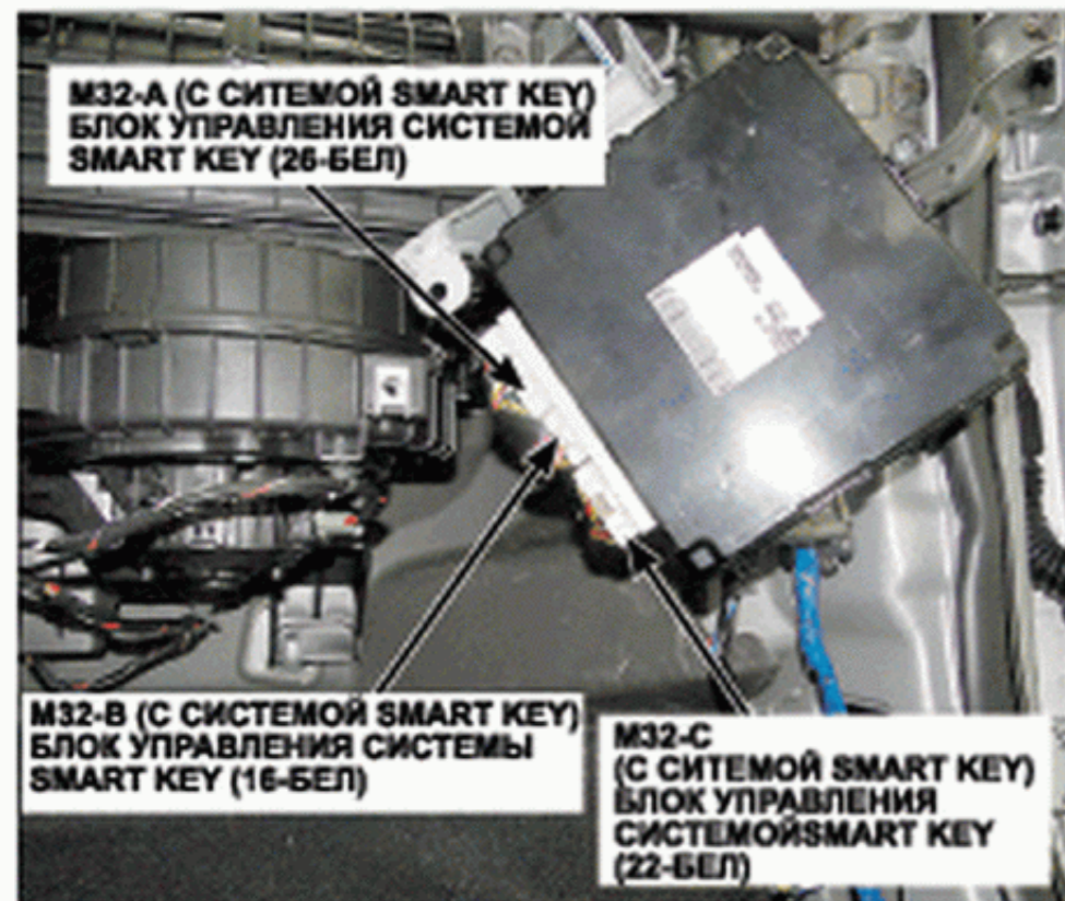
55. Нижняя правая часть панели приборов
