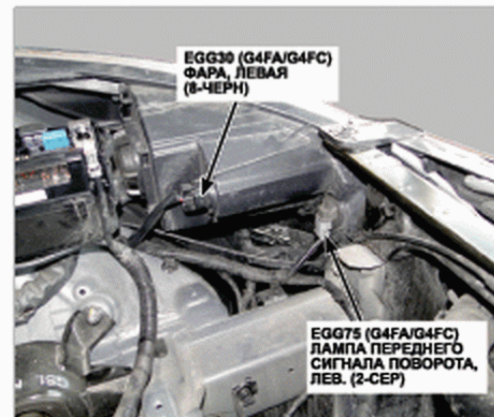
9. Передняя левая часть моторного отсека
