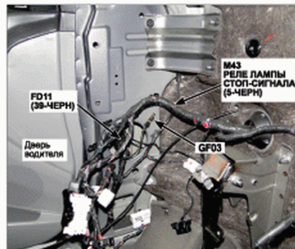
46. Нижняя часть левой передней стойки (кузова)
