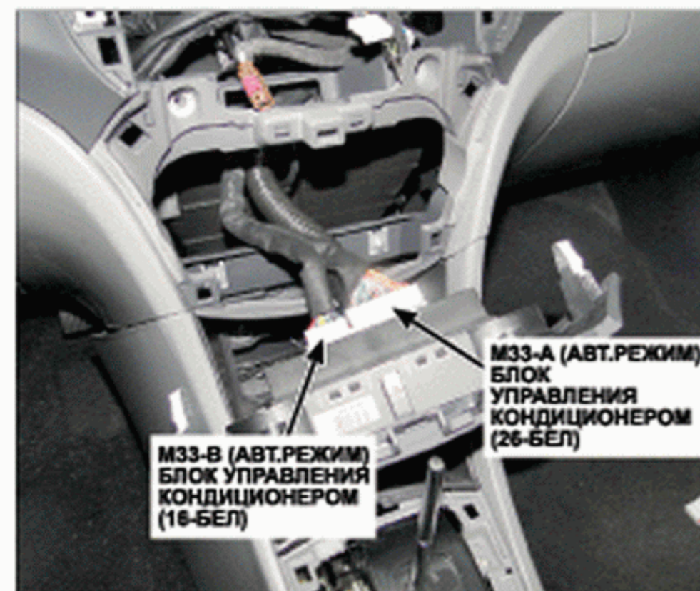
37. Средняя часть панели приборов
