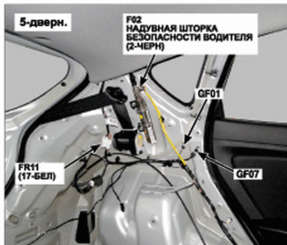
74. Левая сторона панели багажника
