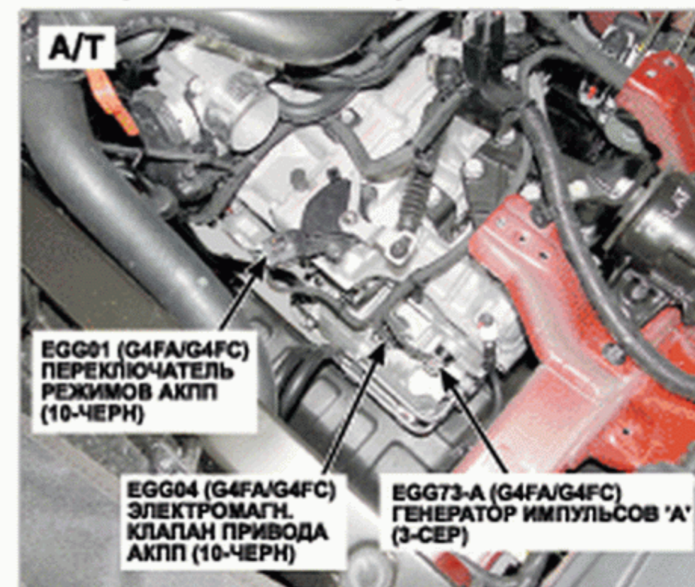
27. Верхняя часть коробки переключения передач
