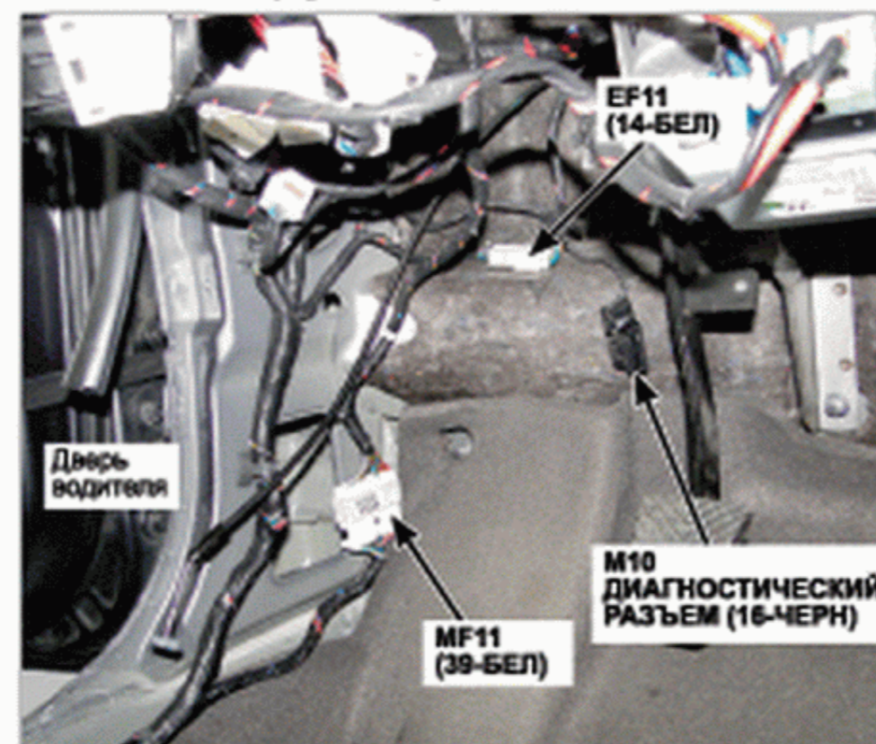
47. Нижняя часть левой передней стойки (кузова)
