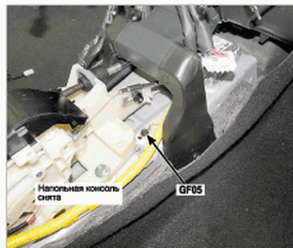
60. Передняя часть консоли
