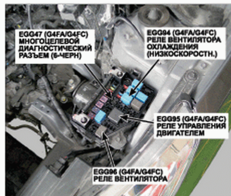
10. Левая сторона моторного отсека
