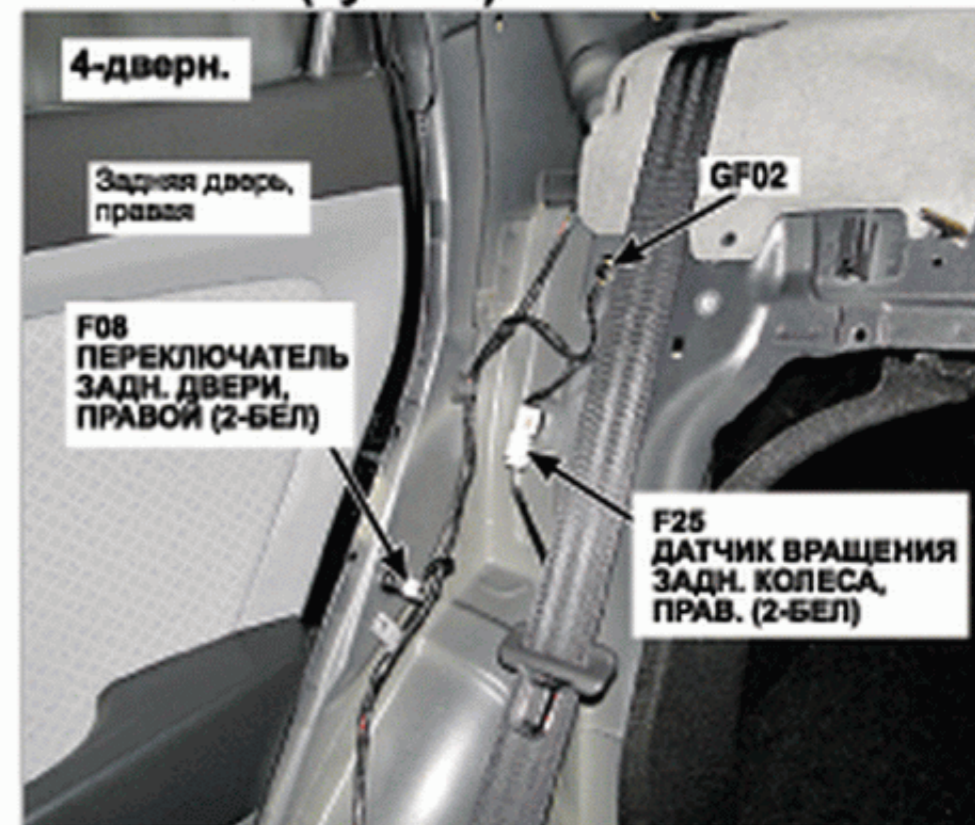
69. Нижняя часть правой задней стойки (кузова)
