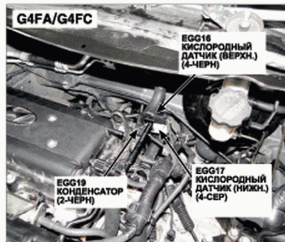
26. Левая сторона двигателя
