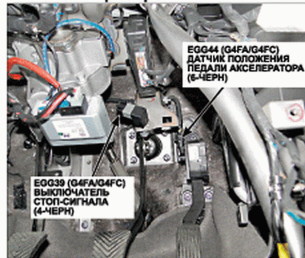
49. Задняя левая часть панели приборов
