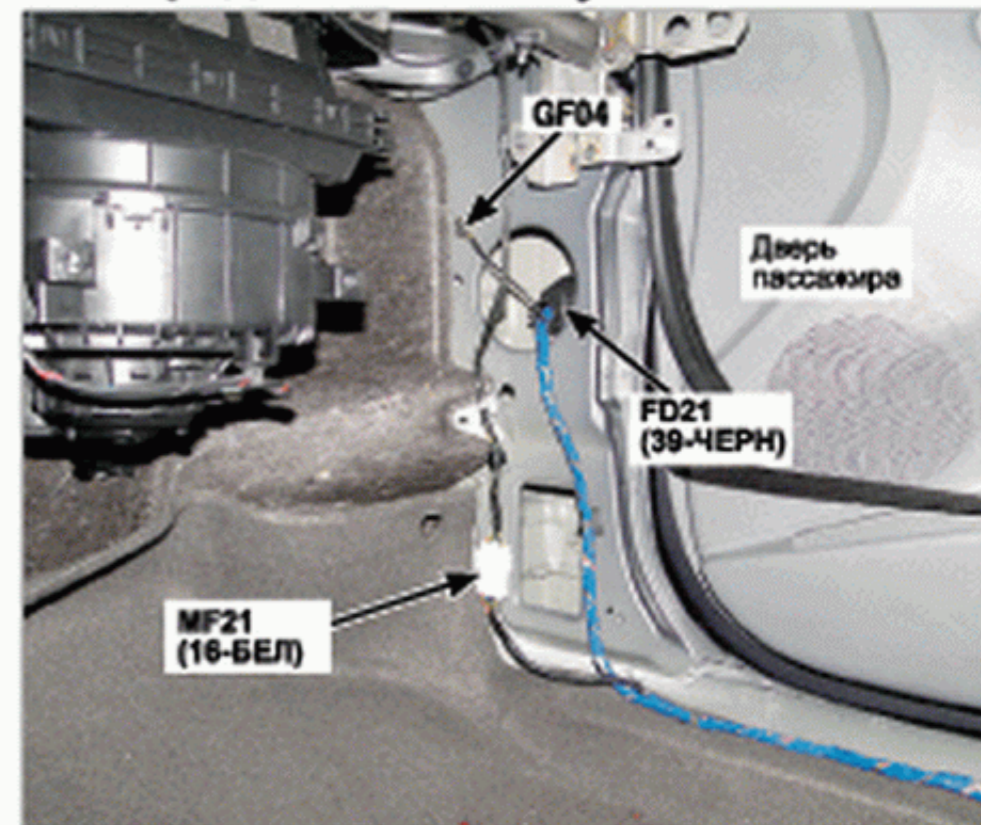
57. Нижняя часть правой передней стойки кузова
