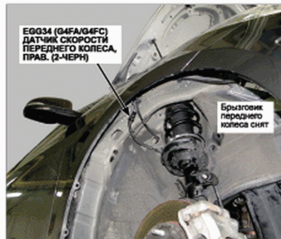
8. Передняя колесная арка, правая
