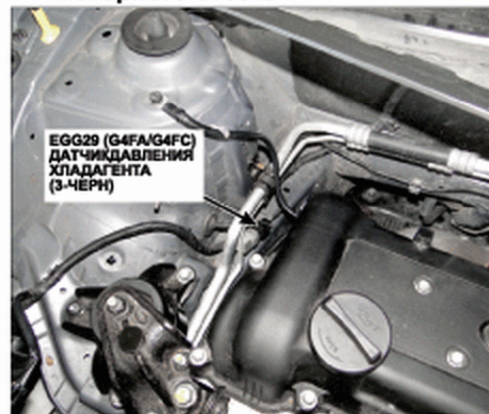
97. Правая задняя часть моторного отсека
