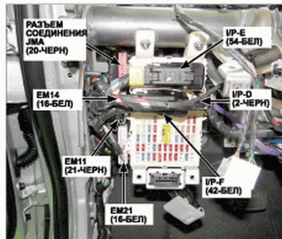
44. Левая сторона панели приборов
