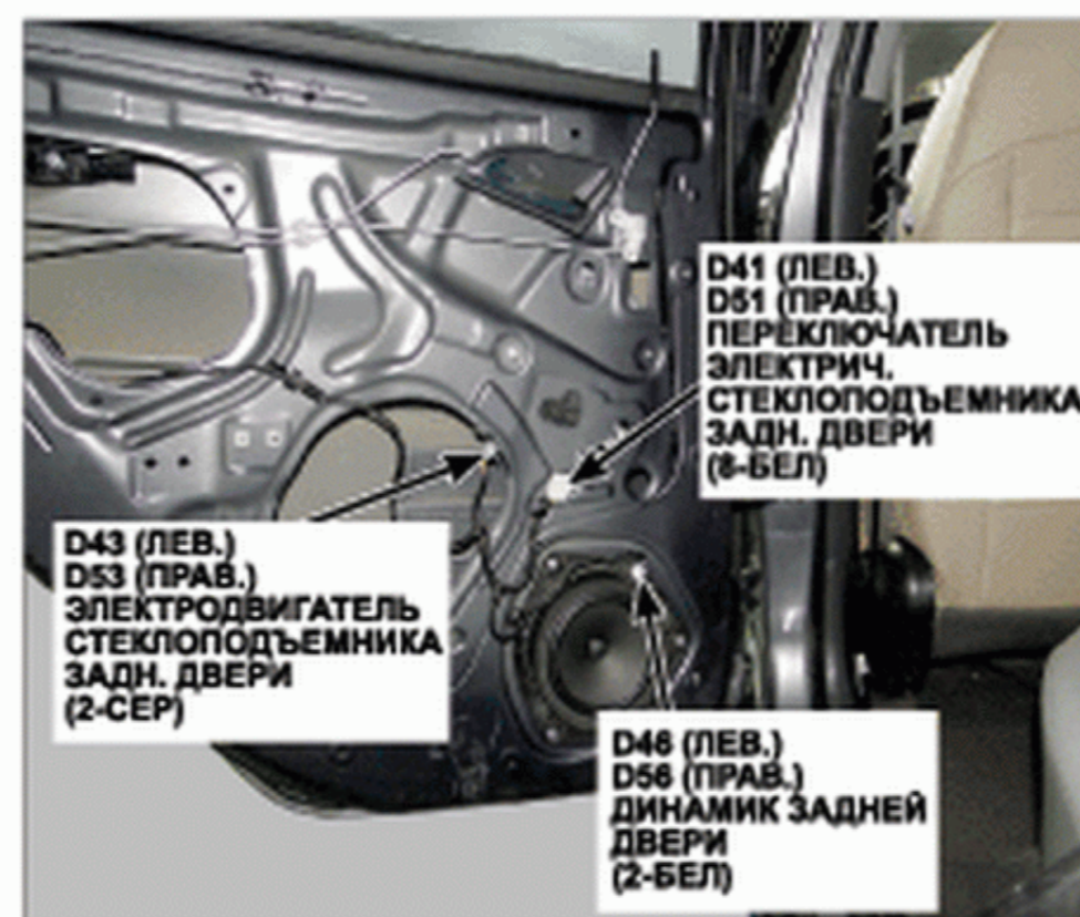
86. Задняя дверь
