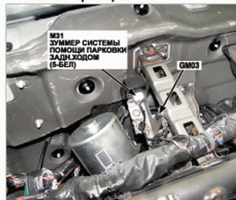
42. Левая верхняя часть панели приборов
