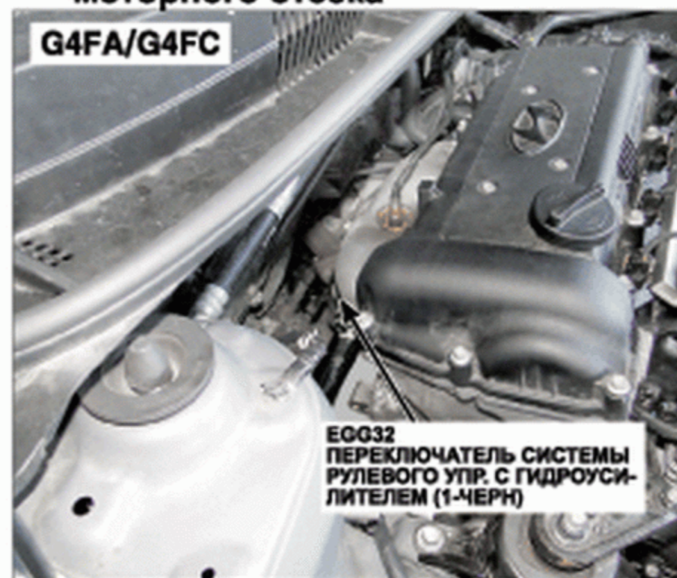
98. Правая задняя часть моторного отсека
