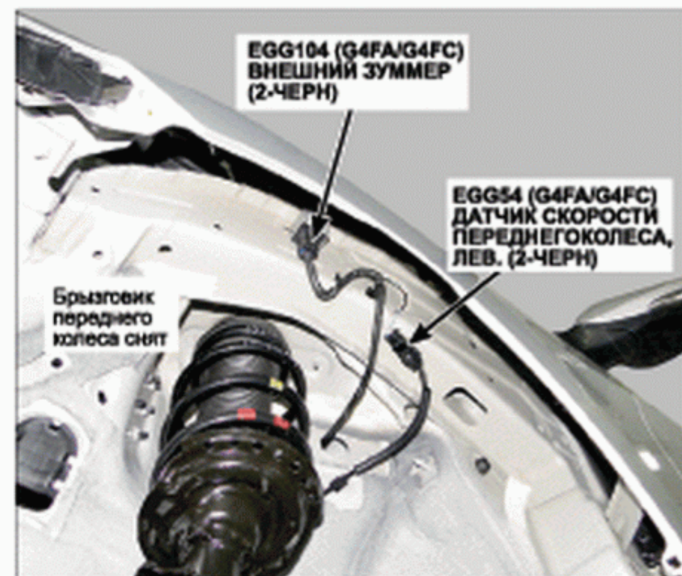
7. Передняя колесная арка, левая
