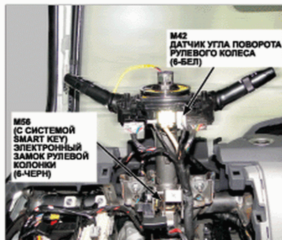
40. Рулевая колонка
