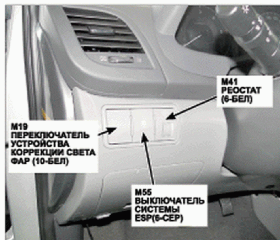
32. Левая сторона панели приборов
