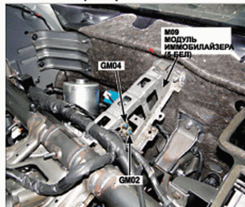
43. Левая верхняя часть панели приборов
