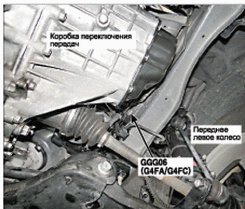
16. Левая сторона моторного отсека
