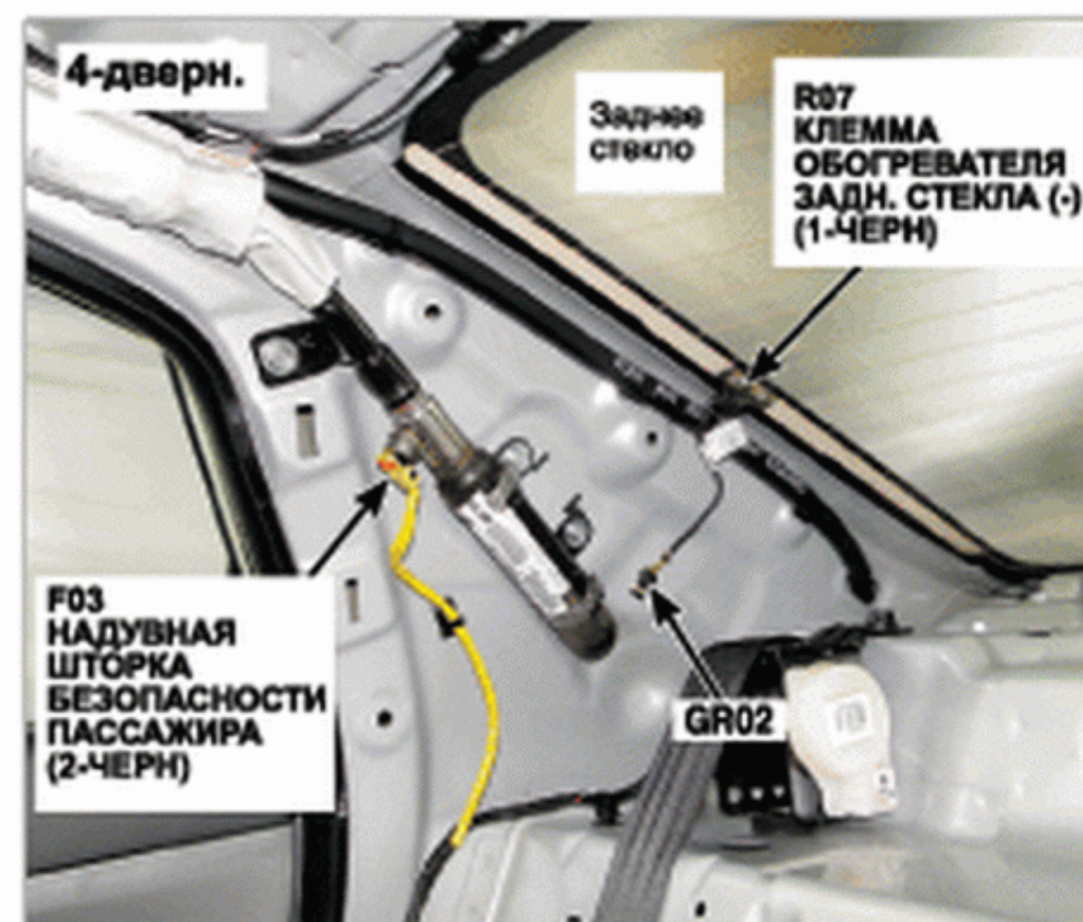
72. Задняя стойка кузова, правая
