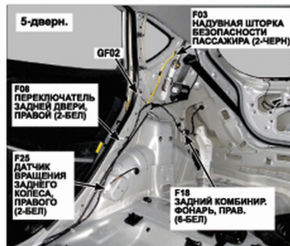
76. Правая сторона панели багажника
