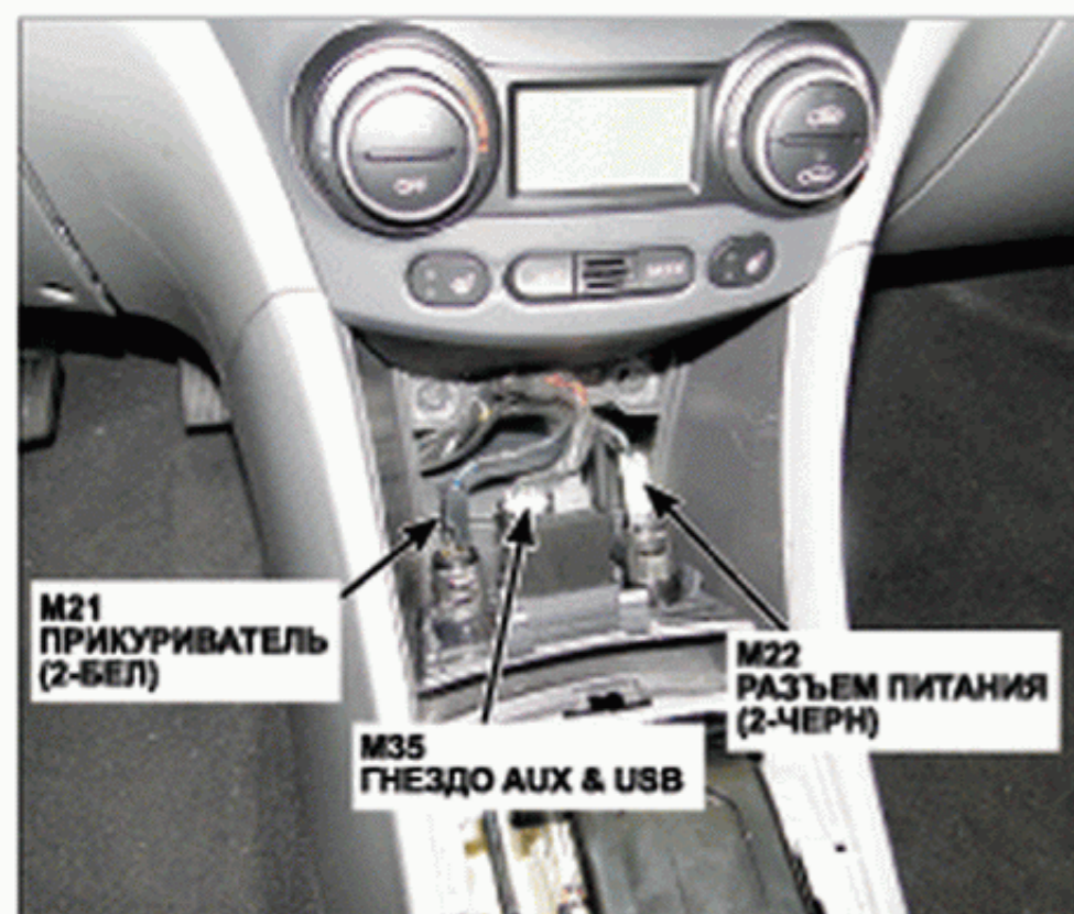
58. Передняя часть консоли
