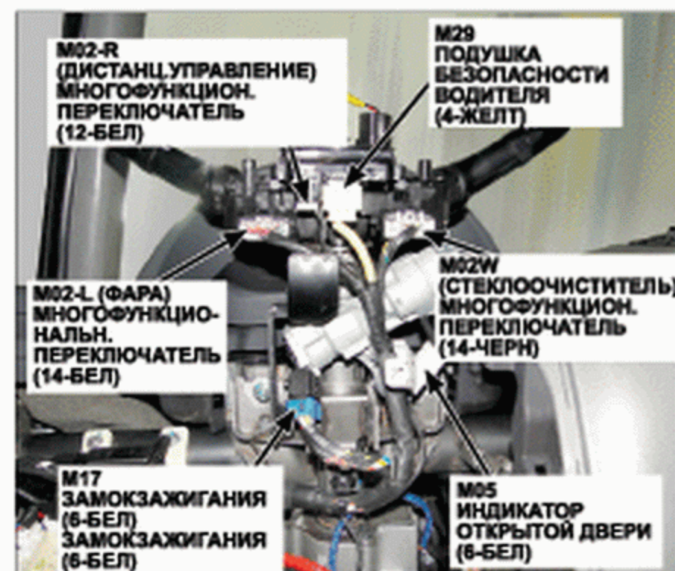
40. Рулевая колонка
