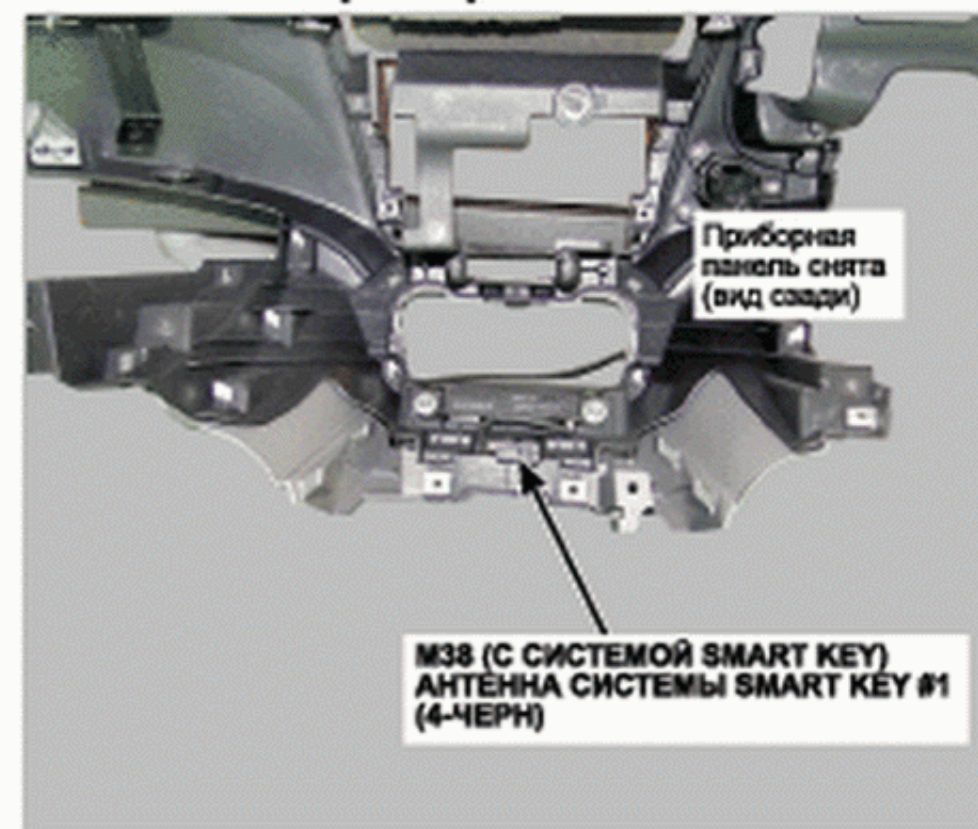
39. Средняя нижняя часть панели приборов
