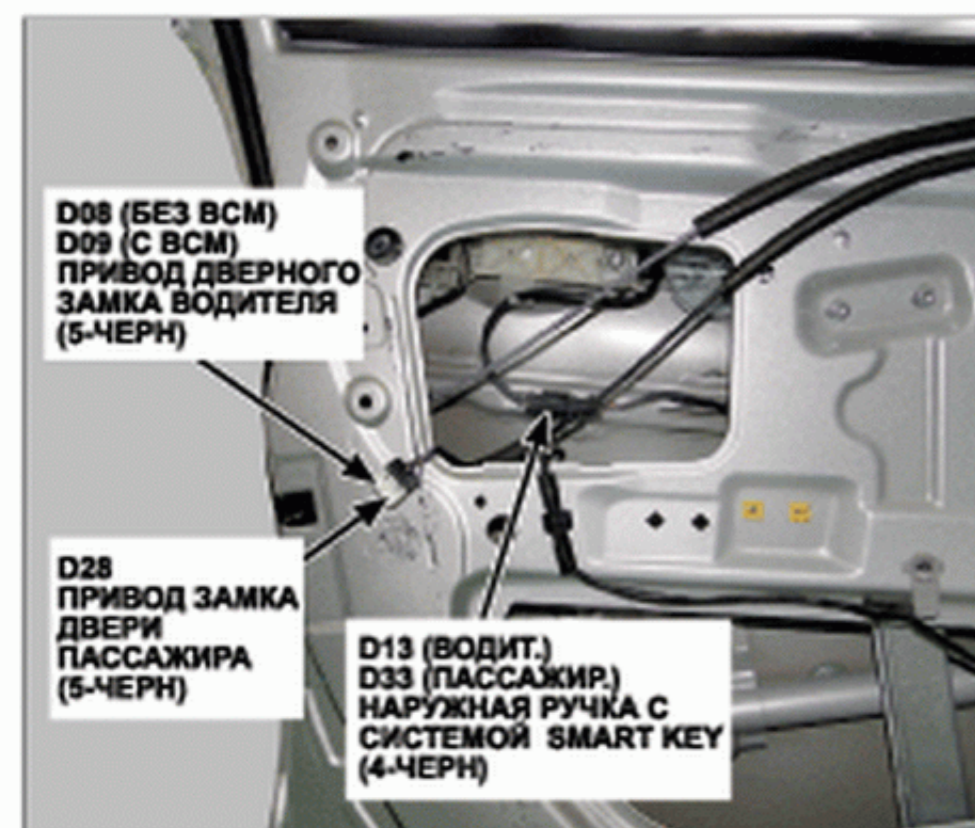
85. Передняя дверь
