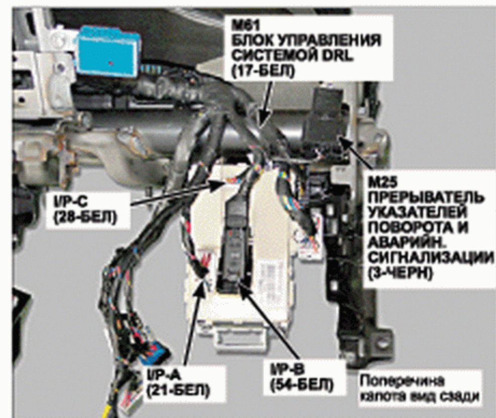
45. Задняя левая часть панели приборов
