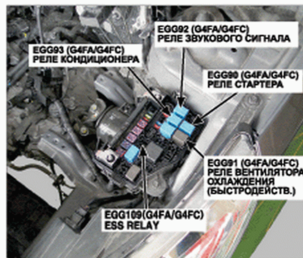
11. Левая сторона моторного отсека
