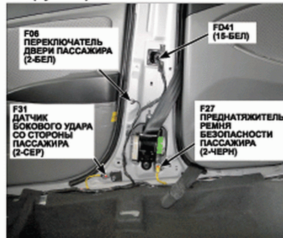
67. Правая центральная стойка (кузова)
