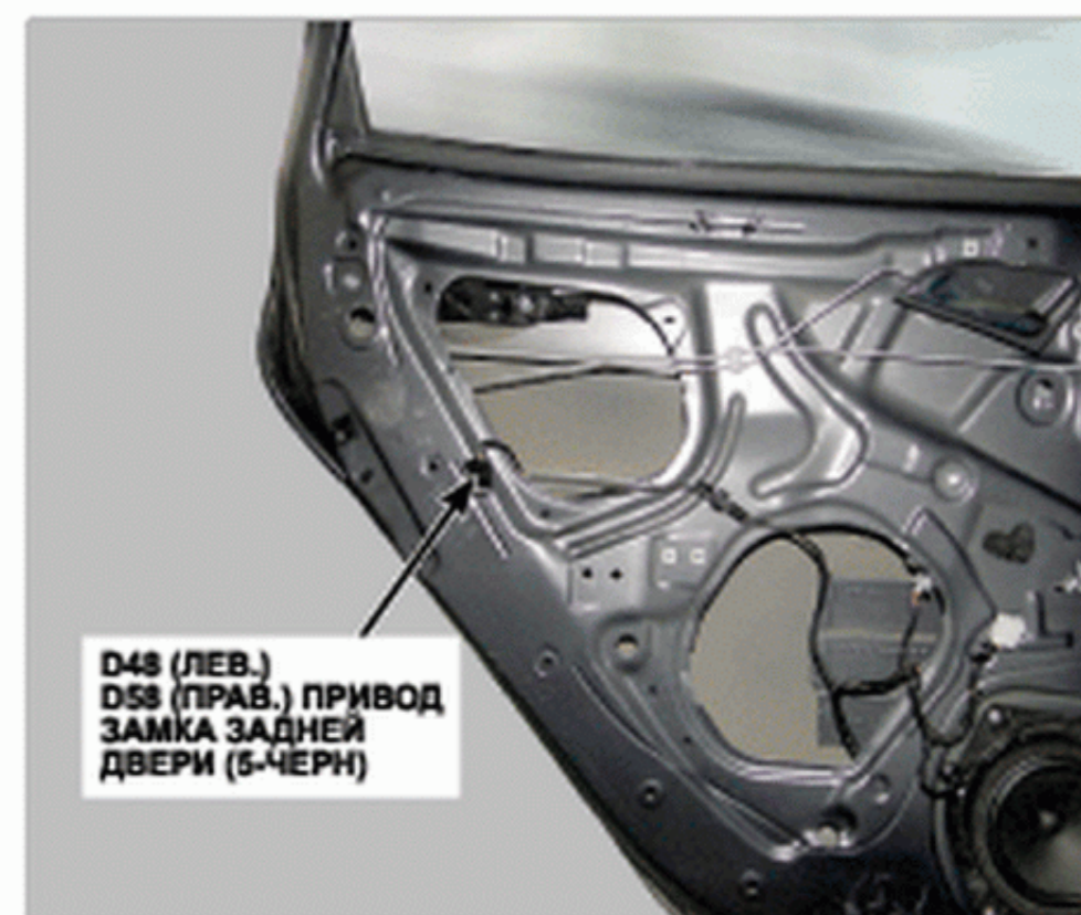
87. Задняя дверь
