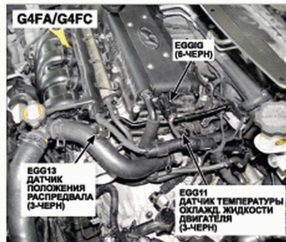
25. Левая сторона двигателя
