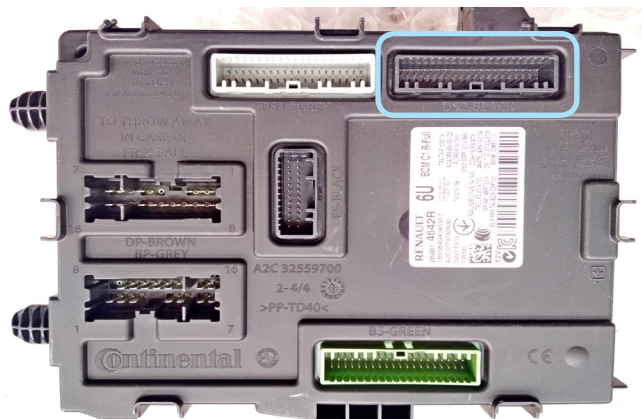
Фото 3.7. Местоположение разъёма на блоке BSI
