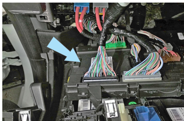
Фото 1.6. Блок BSI снят
