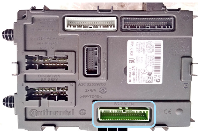
Фото 3.3. Местоположение разъёма на блоке BSI
