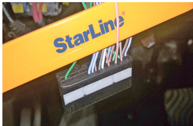
Фото 3.8. Управление системой климат-контроля (розово-белый)
