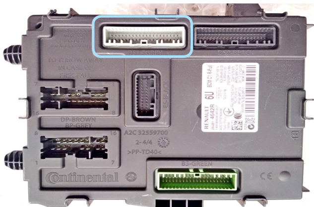
Фото 3.5. Местоположение разъёма на блоке BSI
