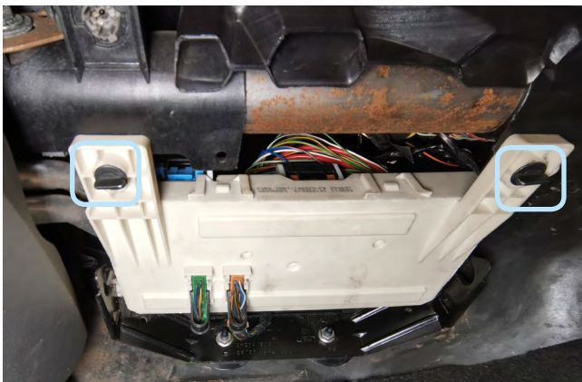
Фото 1.3. Клипсы крепления блока GEM.
