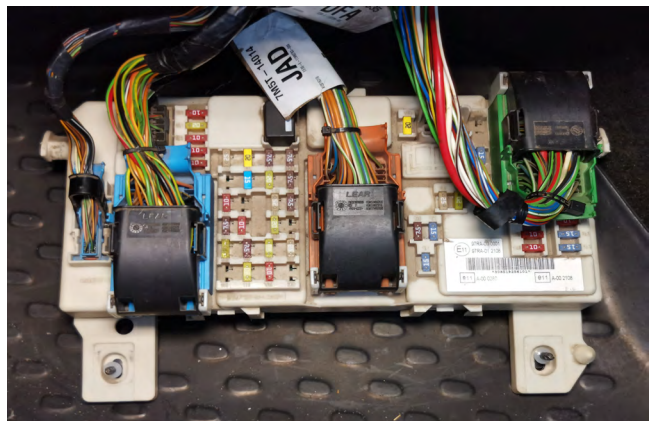
Фото 1.4. Блока GEM снят.
