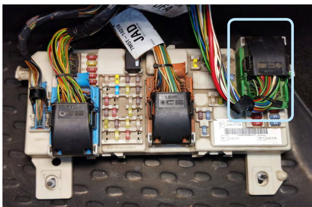
Фото 3.17. Местоположение разъёма С96
