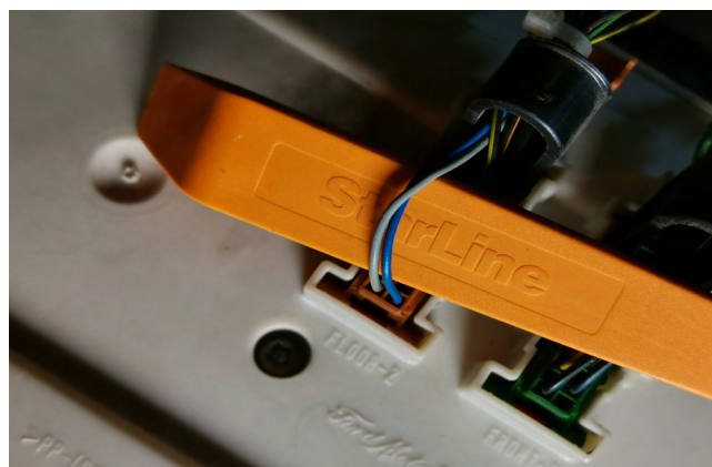
Фото 3.3. Шина CAN-A (серый и синий)
