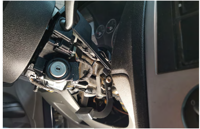
Фото 1.8. Нижняя часть кожуха рулевой колонки снята.
