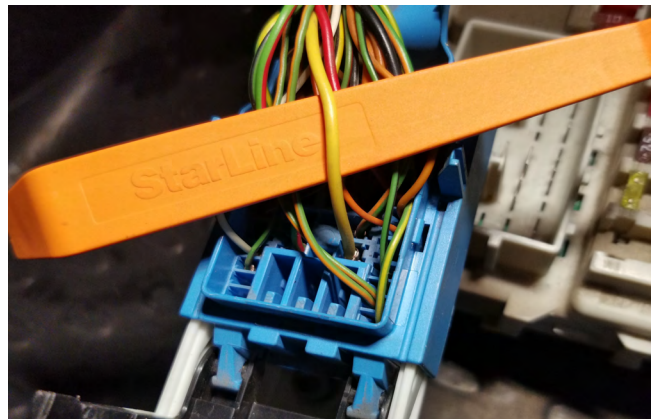
Фото 3.11. Аксессуары (жёлтый)
