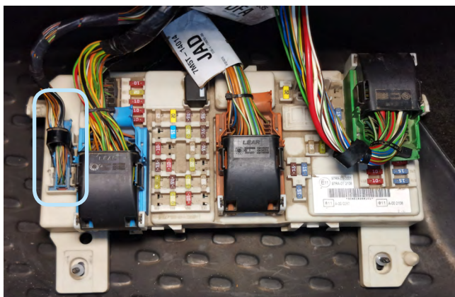
Фото 3.6. Местоположение разъёма С103
