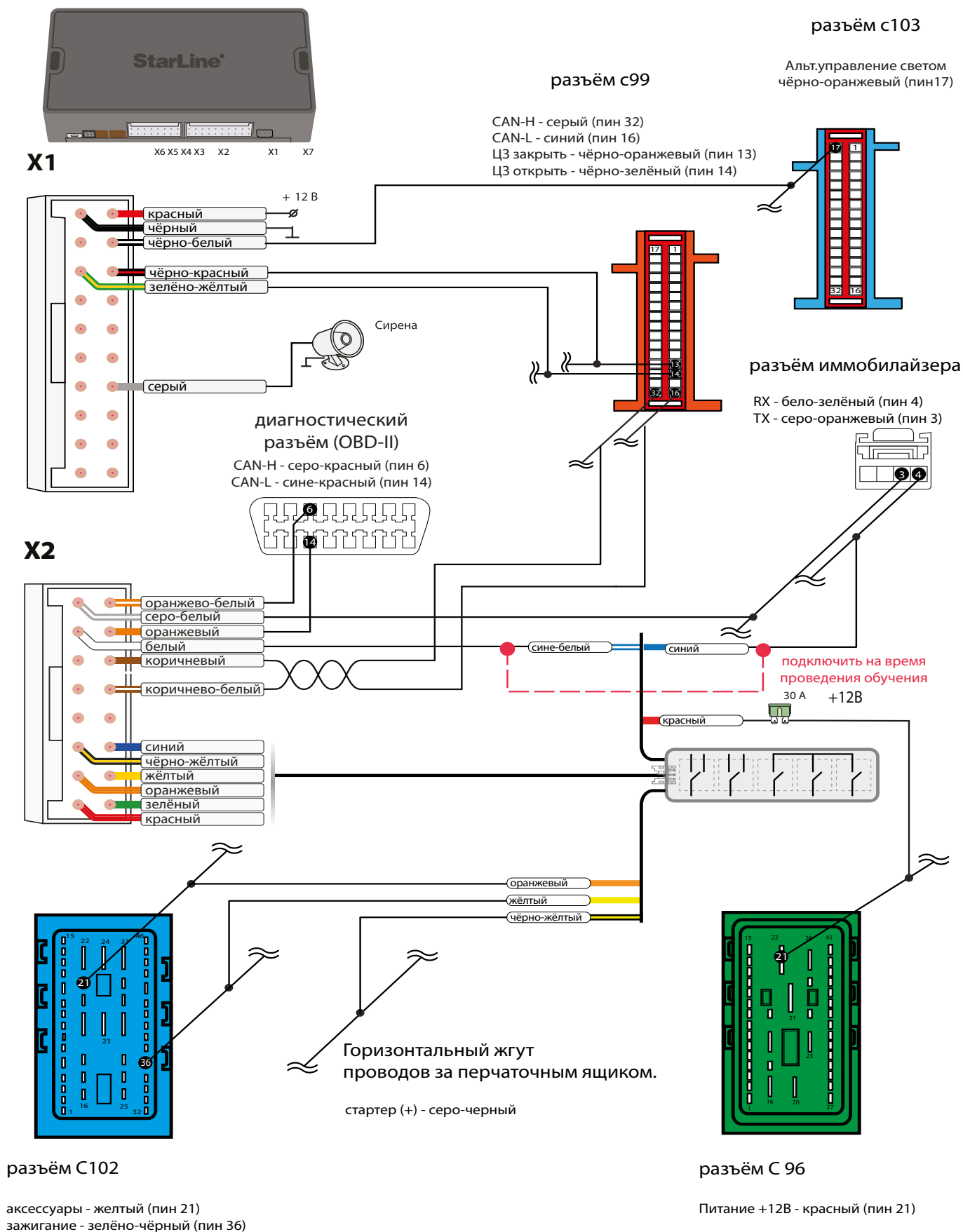
Схема 1. Общая схема подключений.
