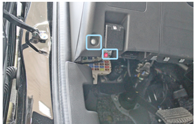
Фото 1.4. Саморезы крепления ручки отпирания лючка топливного бака и пластиковой наклейки
