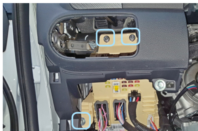
Фото 1.12. Блок кнопок снят. Крепление монтажного блока предохранителей
