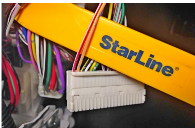
Фото 3.3. Шина CAN-A (жёлто-розовый и красно-белый)
