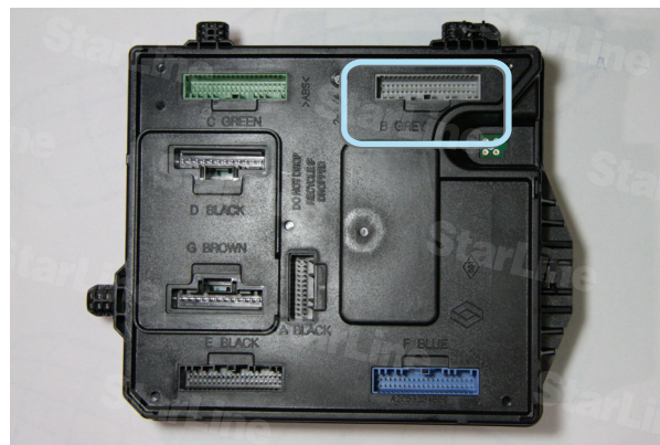
Фото 7.1. Расположение разъема В GREY на центральном коммуникационном блоке салона
