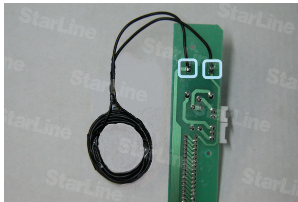
Фото 8.2. Точки пайки изготовленной рамки на плате обходчика BP-03
