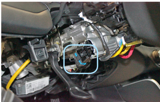
Фото 3.10. Местоположение разъёма
