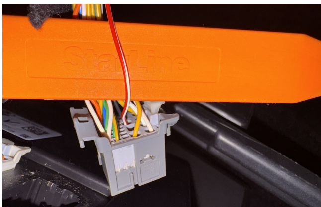
Фото 3.10. Провод управления кнопкой Старт-Стоп
