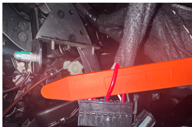
Фото 3.12. Зажигание 1 (красный)
