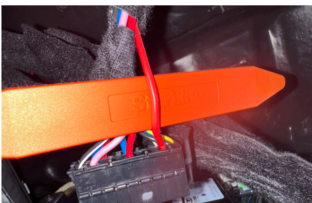
Фото 3.16. Питание +12 (красный)
