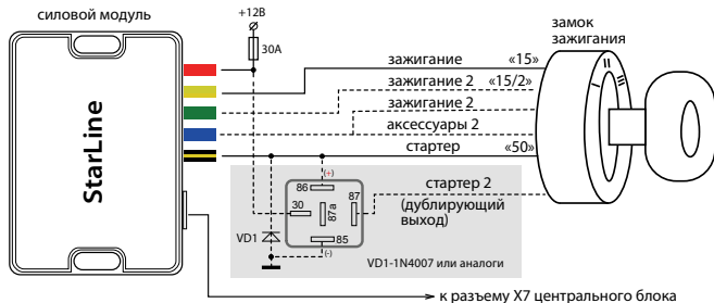
разъем X7 (слаботочные выходы)
